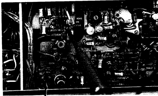
R10 1 MEG LEVEL ZERO Adj.
