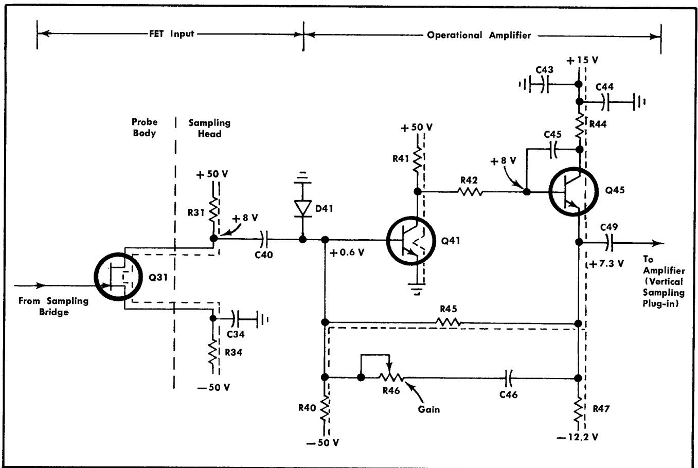
Fig. 3-4. Preampifier circuit.
