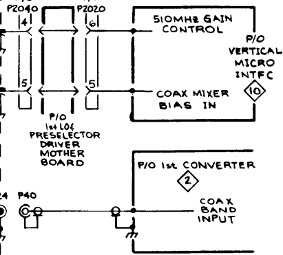
A2690 510MHz IF AMPLIFIER
