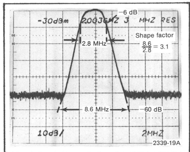
Fig. 4-5. Display Mode 10 dB/DIV.
