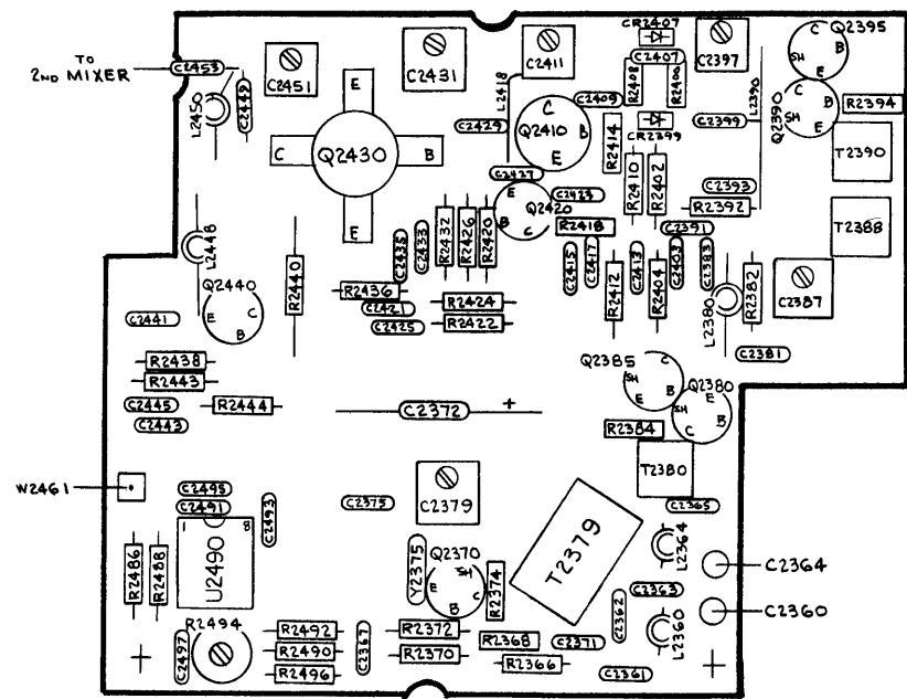
7L18 H-5033-02 A2360A1 500MHz LO
