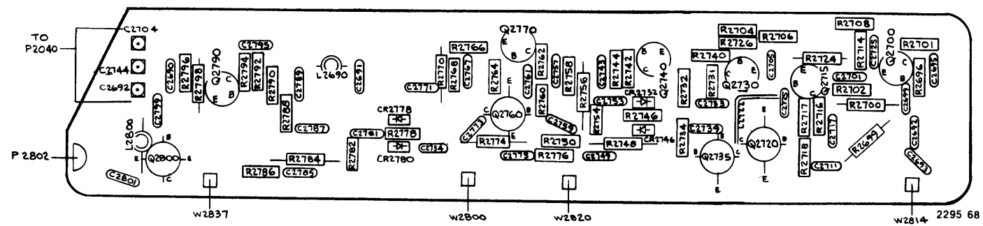
7L18 H-5038-01 A2690A1 510MHz AMPLIFIER
