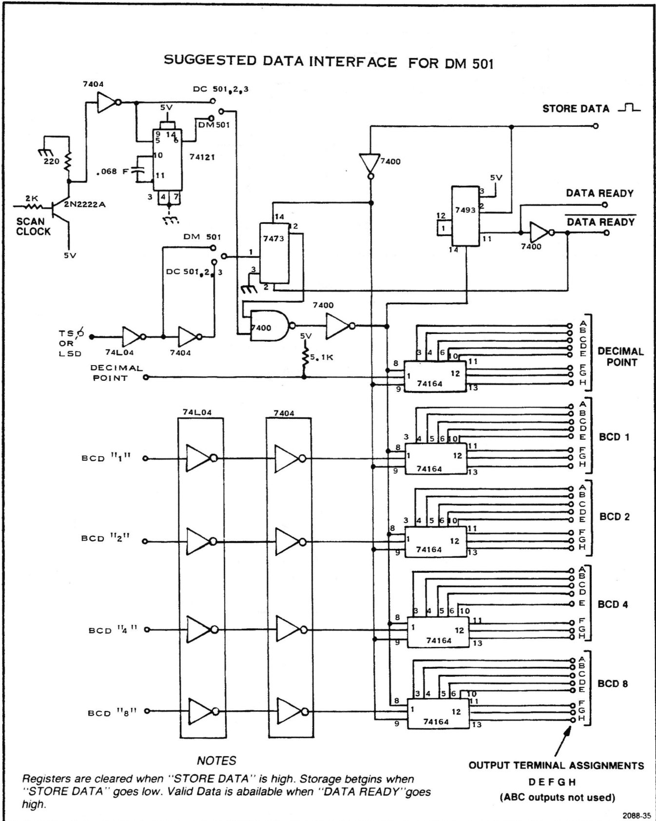
Fig. DM 501-4. Data interface.
